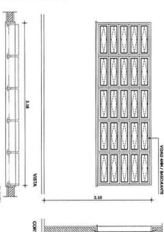
08 | PAGINAÇÃO JANELA J8
