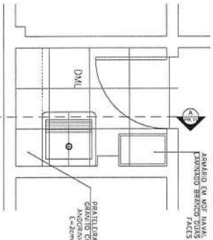
05 PLANTA BAIXA - DML Esc. 1/20
