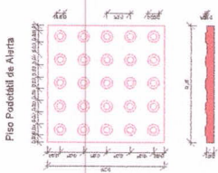
DET. PISO PODOTÁTIL 1:5
